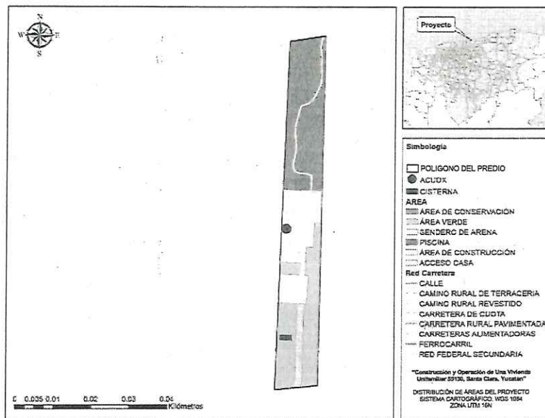
Figura 1. Mapa del diseño del proyecto después de la modificación.
