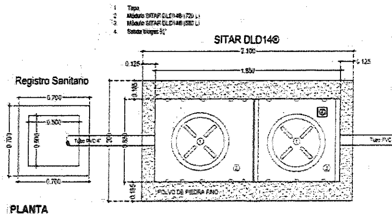
Figura 5.- Planta arquitectónica sugerida para la instalación del SITAR DLD14.
