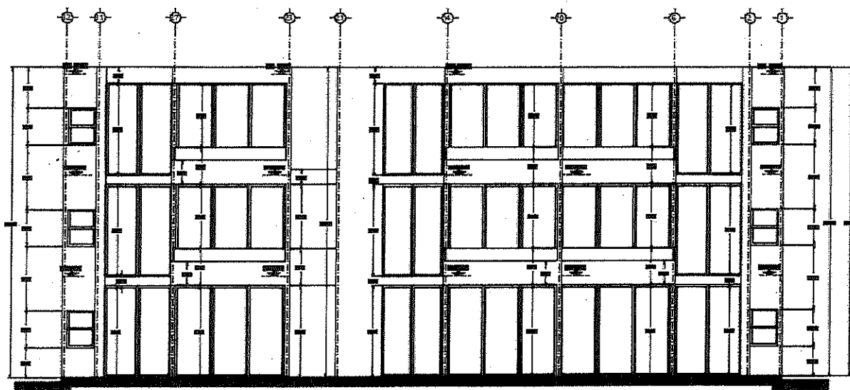
FACHADA FRONTAL
