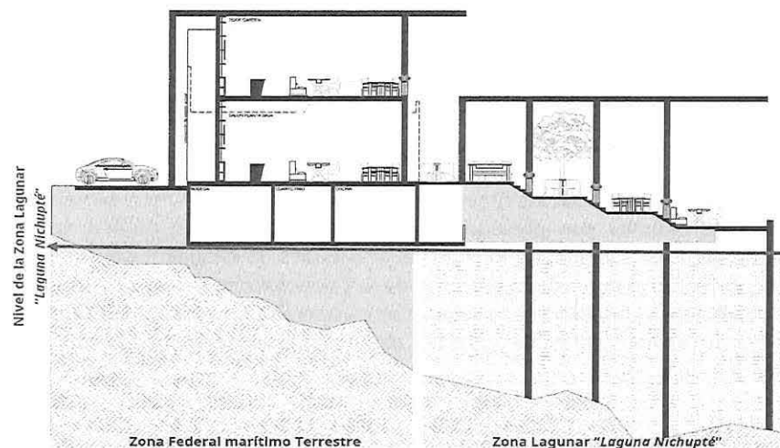
Imagen 3. Corte longitudinal del Proyecto , en el que se observa la intervención de la Zona Lagunar, presentado por la Promovente .
